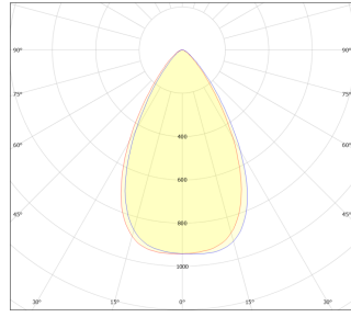
60 Derece Lens / 60 Degree
