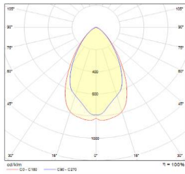
Işık Dağılımı / Light Distribution
