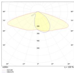
Işık Dağılımı / Light Distribution
