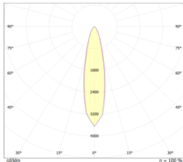
Işık Dağılımı / Light Distribution
